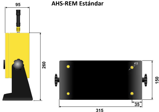
Versión 220 Vca
